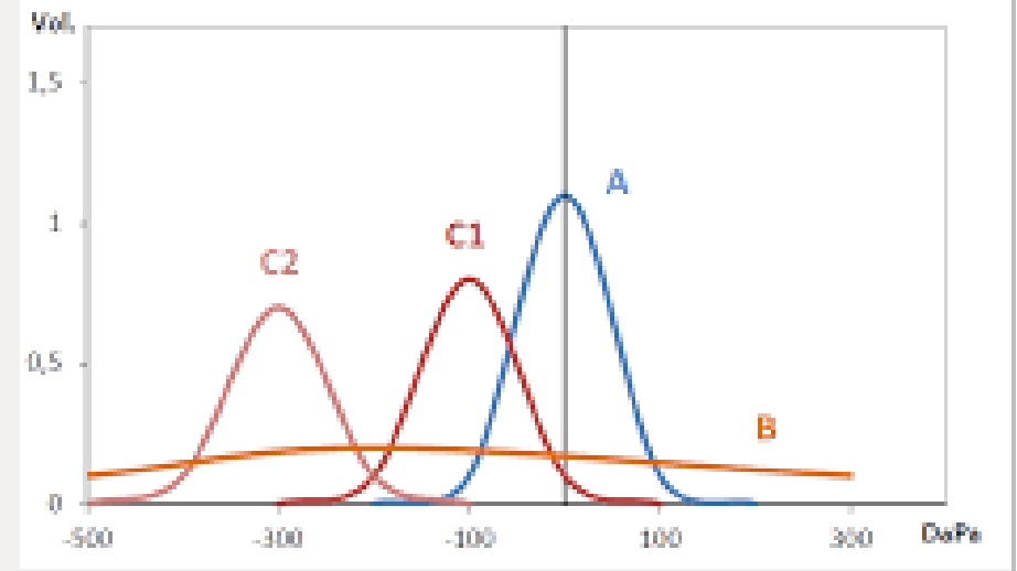
Tympanometri: B-kurve.
